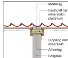
Figur 13 – Brandkarmserstatning under tag med tegl
