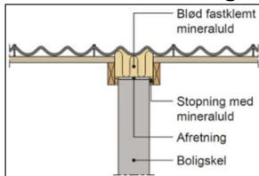
Figur 12 – Brandkarmserstatning under tag med bølgeplader.
