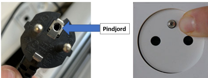
Stikprop med sidejord og pindjord samt en stikkontakt med pindjord
