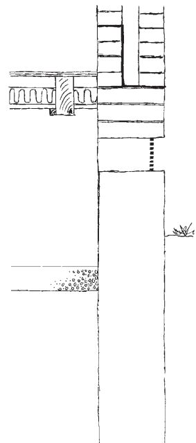
Krybekælder, gulv af træ
