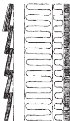
Klinkerbeklædt træskeletvæg
